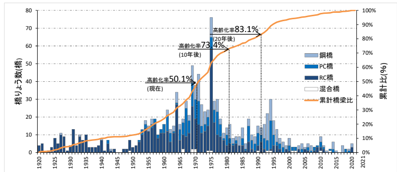
図 建設年別の県管理橋りょう数の分布（令和3年3月）
